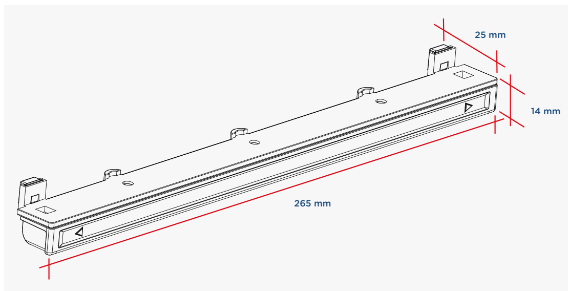
Überschlagslüfter ÜL
